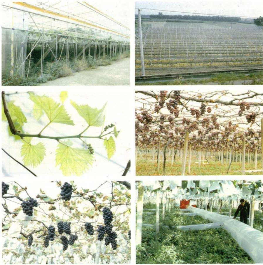
圖 1. 半邊屋頂式結構之設施葡萄簡易溫室
