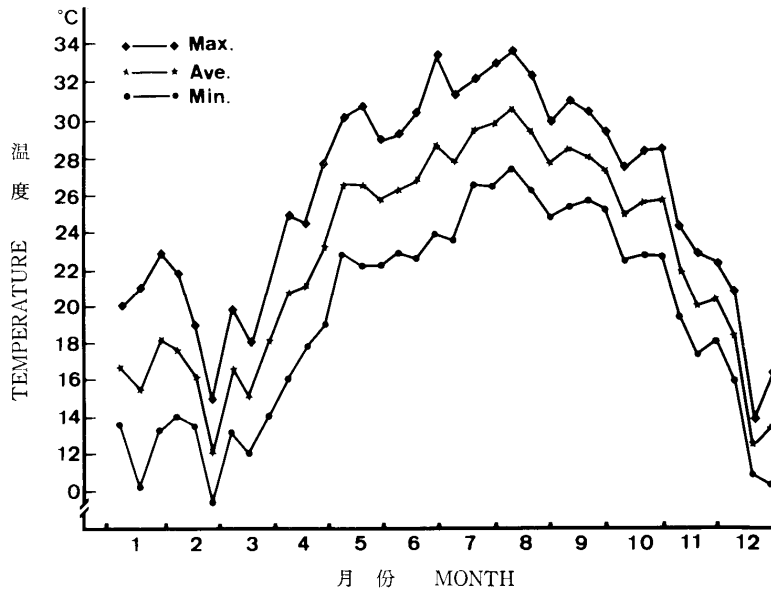
圖 3. 1985 年臺灣中部各旬平均氣溫變化
